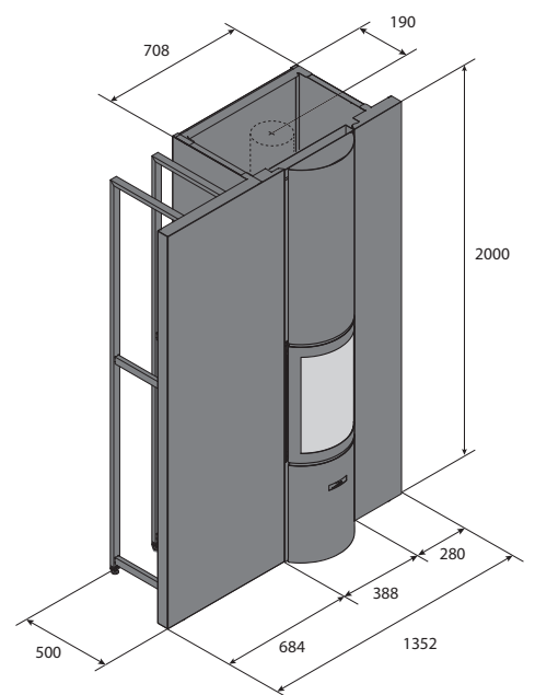
Stův 30-compact in křivé vložky s opláštěním
