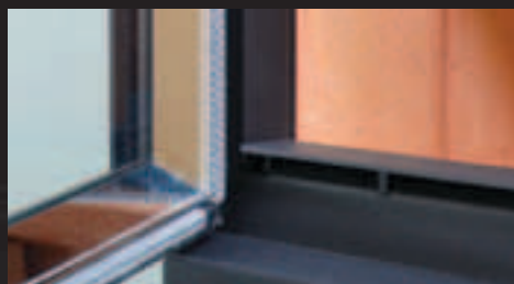
vnútorná kotviaca a tesniaca časť/nerez
