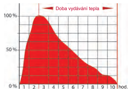
Doba vydávání tepla po 3 vkladkách dřeva vždy po 2 kg
